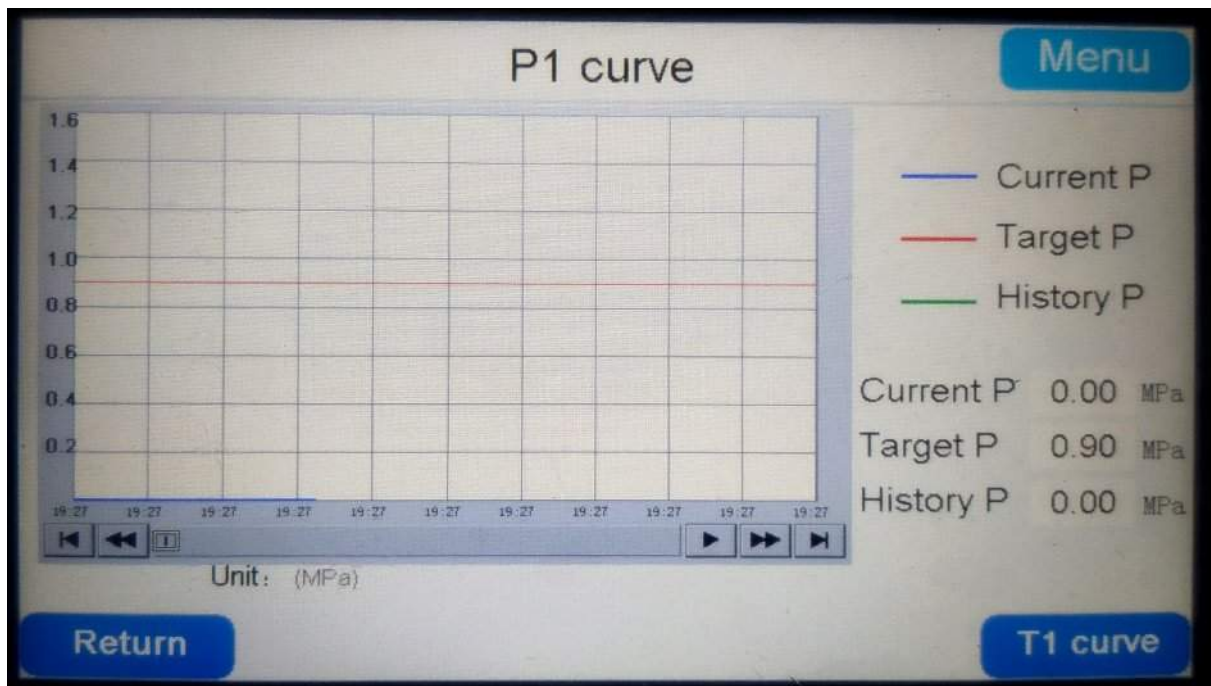
Saspiesta gaisa spiediena līkne darbības laikā.
